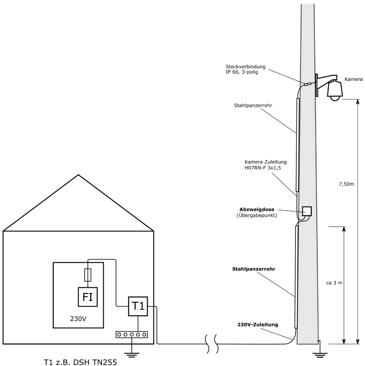
Abbildung 1: Installationsskizze des Kamerasystems
